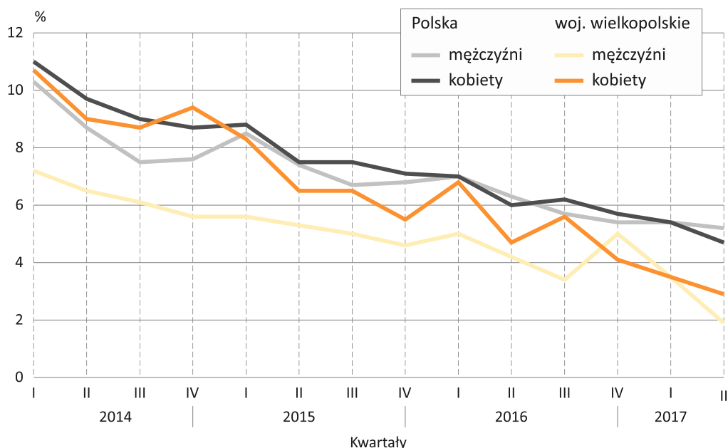
Ryc. 8. STOPA BEZROBOCIA
