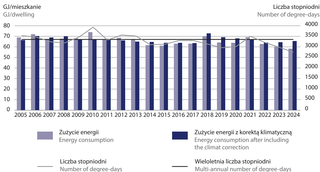
Wykres 22. Zużycie energii w gospodarstwach domowych w przeliczeniu na 1 mieszkanie
