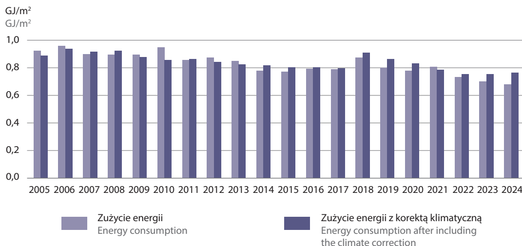
Wykres 23. Zużycie energii w gospodarstwach domowych w przeliczeniu na 1 m 2 powierzchni mieszkania Chart 23. Residential energy consumption per 1 m 2 of dwelling area
