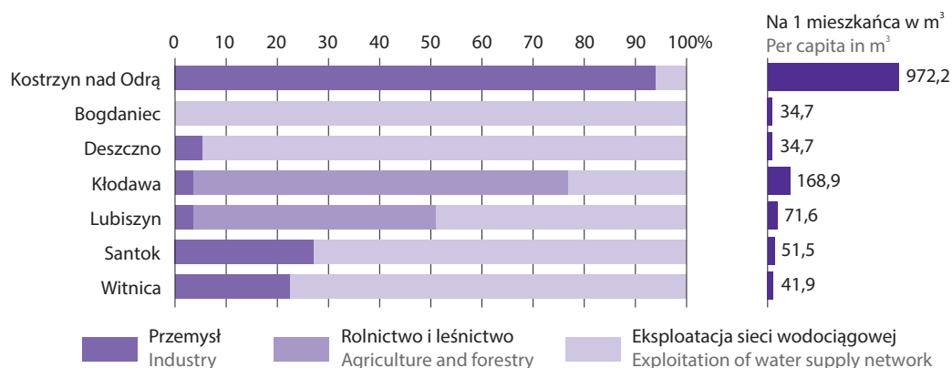
Wykres 1. Zużycie wody na potrzeby gospodarki narodowej i ludności w 2024 r. Chart 1. Water consumption for needs of the national economy and population in 2024
