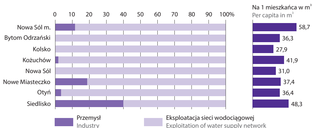
Wykres 67. Zużycie wody na potrzeby gospodarki narodowej i ludności w 2024 r. Chart 67. Water consumption for needs of the national economy and population in 2024
