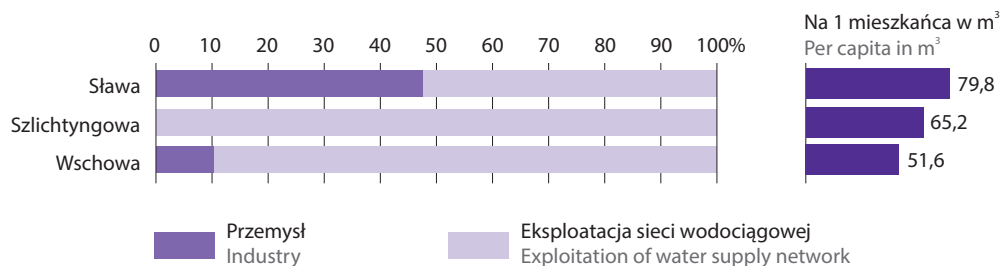
Wykres 164. Zużycie wody na potrzeby gospodarki narodowej i ludności w 2024 r. Chart 164. Water consumption for needs of the national economy and population in 2024
