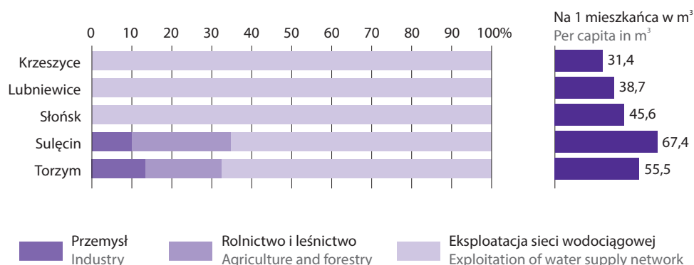
Wykres 127. Zużycie wody na potrzeby gospodarki narodowej i ludności w 2024 r. Chart 127. Water consumption for needs of the national economy and population in 2024
