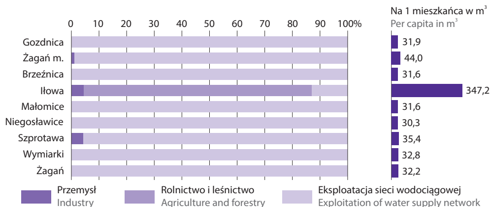
Wykres 204. Zużycie wody na potrzeby gospodarki narodowej i ludności w 2024 r. Chart 204. Water consumption for needs of the national economy and population in 2024
