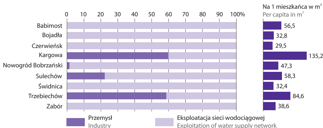
Wykres 175. Zużycie wody na potrzeby gospodarki narodowej i ludności w 2024 r. Chart 175. Water consumption for needs of the national economy and population in 2024
