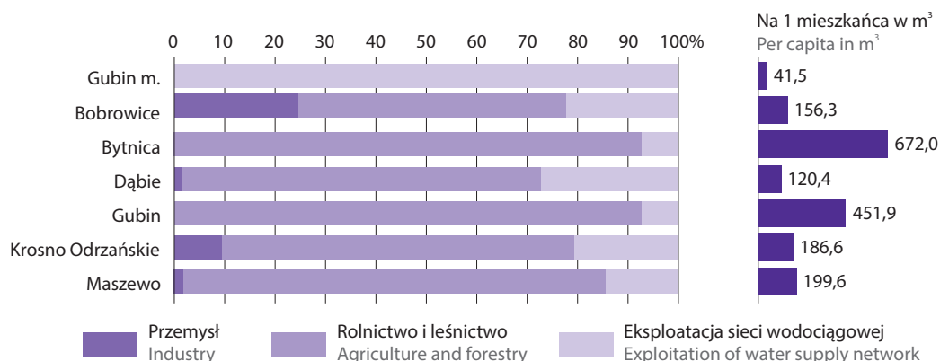
Wykres 24. Zużycie wody na potrzeby gospodarki narodowej i ludności w 2024 r. Chart 24. Water consumption for needs of the national economy and population in 2024
