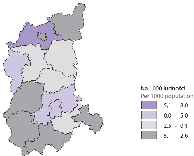
Mapa 4. Saldo migracji na pobyt stały w 2024 r. Map 4. Net migration for permanent residence in 2024
