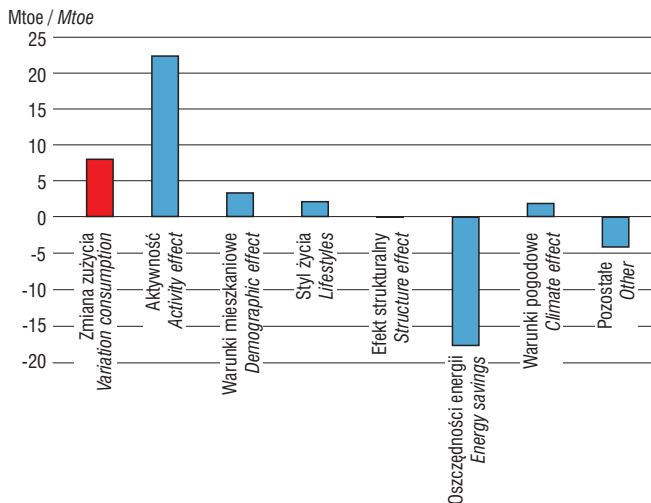
Zużycie energii pierwotnej w latach 2000–2013 – wpływ czynników Primary energy consumption in years 2000–2013 – driving factors
