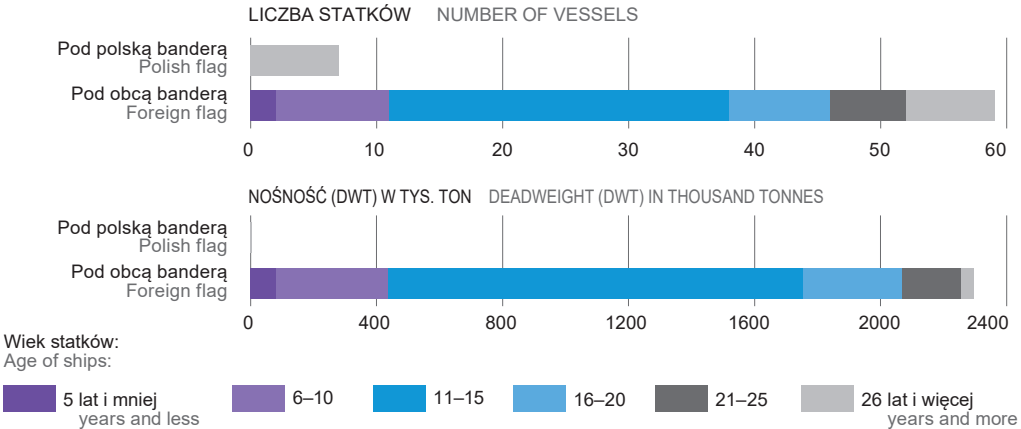
WYKRES 6 (107). MORSKA FLOTA TRANSPORTOWA WEDŁUG WIEKU STATKÓW W 2023 R. CHART 6 (107). MARITIME CARGO-CARRYING FLEET BY AGE OF SHIPS IN 2023
