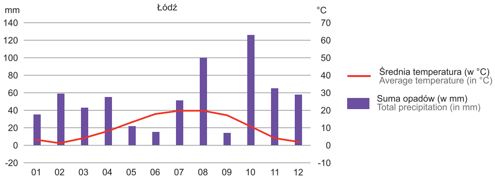
WYKRES 1. TEMPERATURY POWIETRZA I OPADY ATMOSFERYCZNE W WYBRANYCH STACJACH METEOROLOGICZNYCH W 2023 R. CHART 1. AIR TEMPERATURES AND ATMOSPHERIC PRECIPITATION IN SELECTED METEOROLOGICAL STATIONS IN 2023
