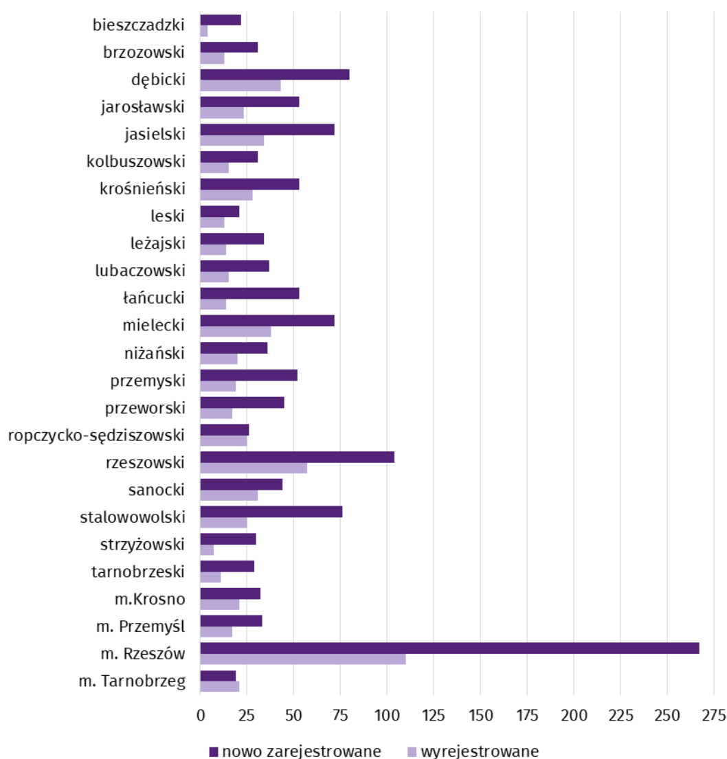
Wykres 10. Podmioty gospodarki narodowej nowo zarejestrowane i wyrejestrowane w maju 2022 r.
