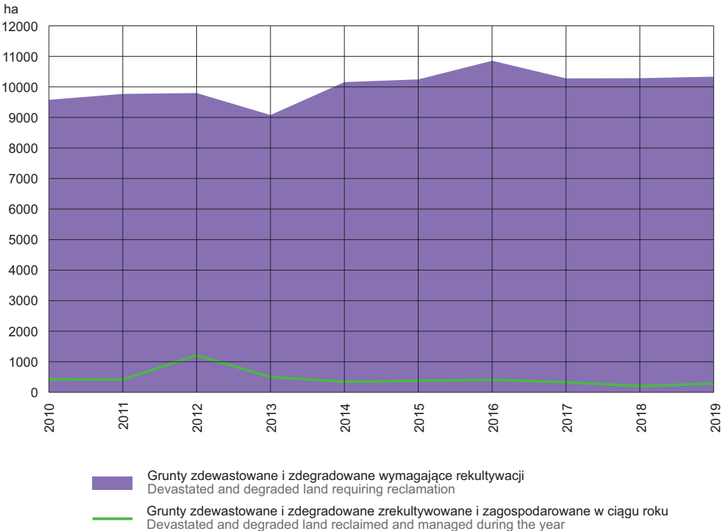
WYKRES 2. GRUNTY ZDEWASTOWANE I ZDEGRADOWANE WYMAGAJĄCE REKULTYWACJI I ZAGOSPODAROWANIA ORAZ GRUNTY ZREKULTYWOWANE I ZAGOSPODAROWANE
