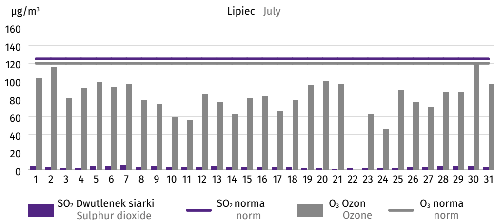
Wykres 33. Miesięczne wyniki automatycznych pomiarów jakości powietrza w III kwartale 2019 r. Chart 33. Monthly results of automatic air quality measurement in the III quarter of 2019
