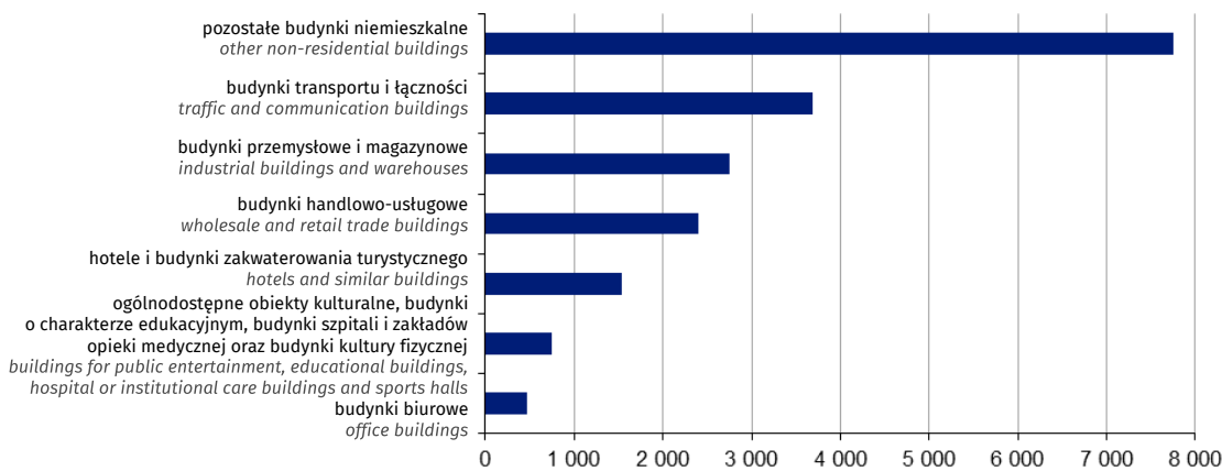
Wykres 16. Liczba nowych budynków niemieszkalnych oddanych do użytkowania w 2024 r. według grup PKOB Chart 16. Number of new non-residential buildings completed in 2024 by groups of PKOB
