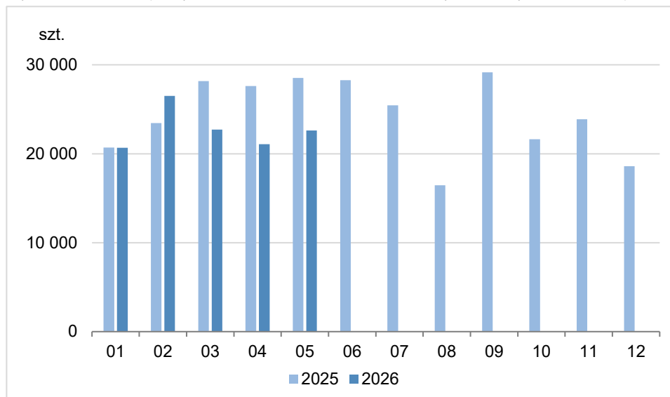
Wykres 2. Produkcja wytworzona silników spalinowych do pojazdów mechanicznych
